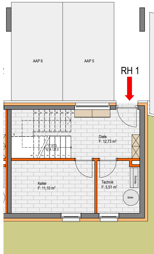
UNTERGESCHOSS
