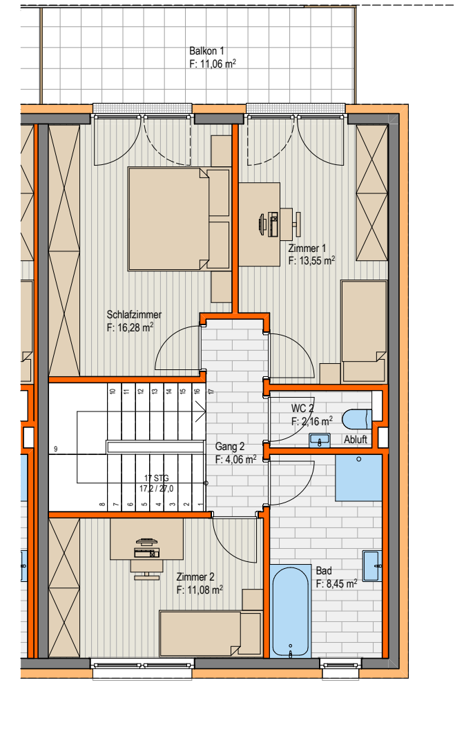
OBERGESCHOSS
