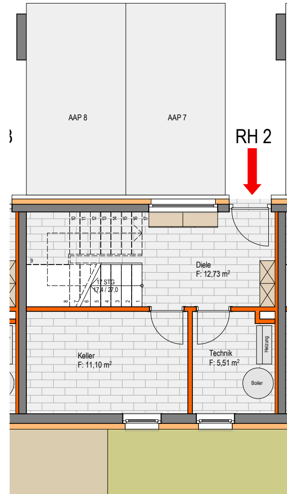
UNTERGESCHOSS
