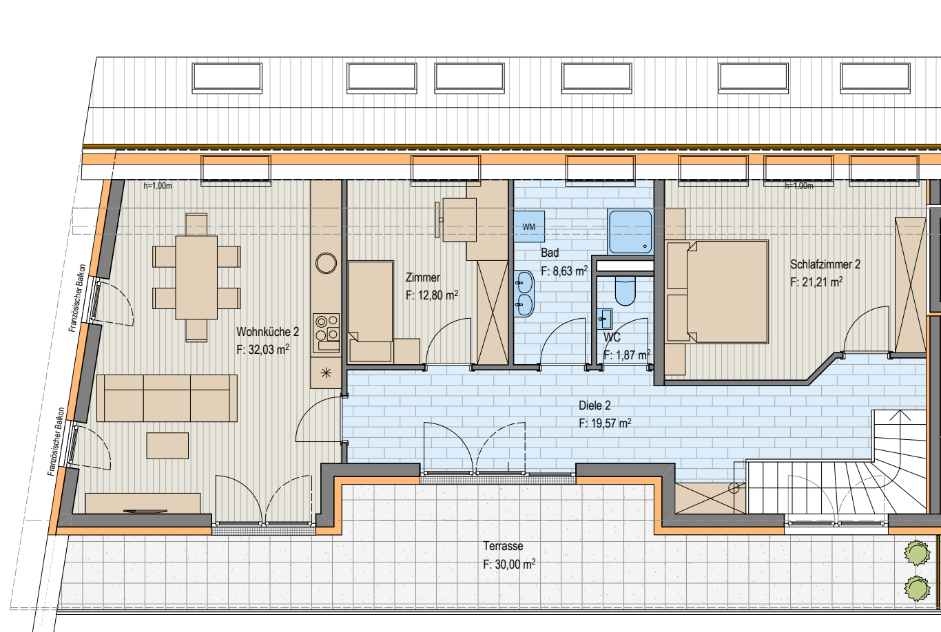
DACHGESCHOSS
