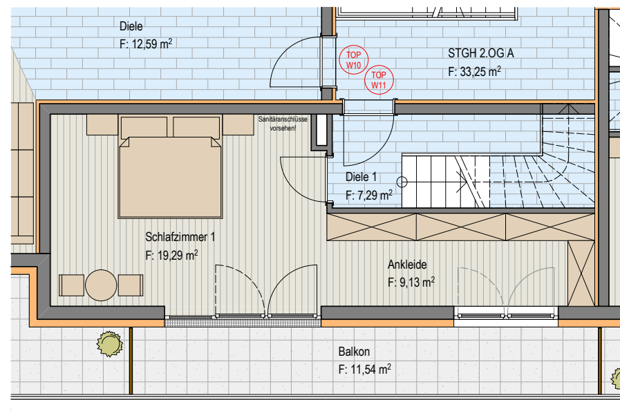
2. OBERGESCHOSS
